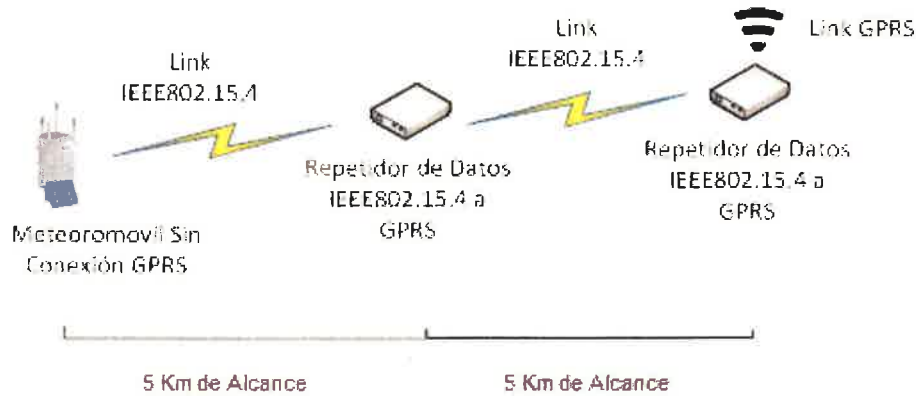
Figura 3 – Diseño conceptual de comunicaciones con repetidores de datos.
