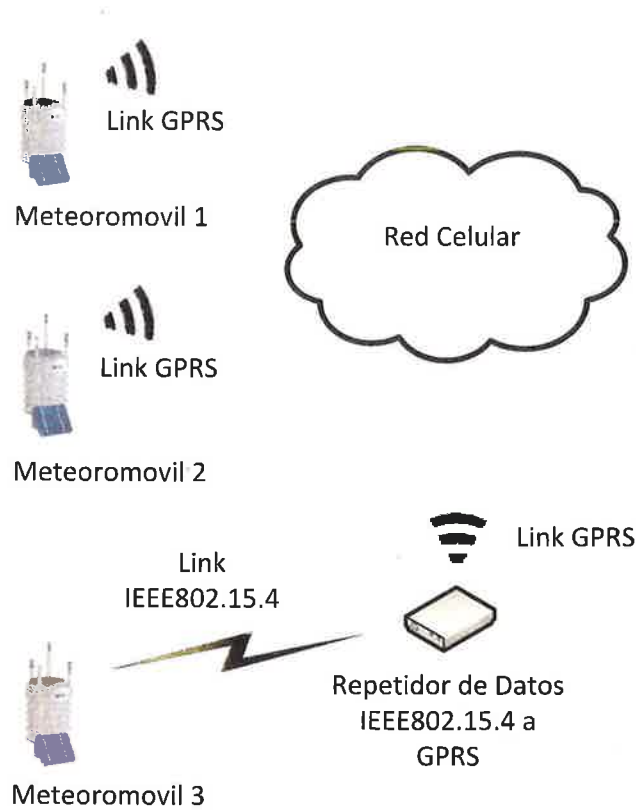
Figura 2 – Diseño conceptual preliminar del proyecto Meteoromóvil.
