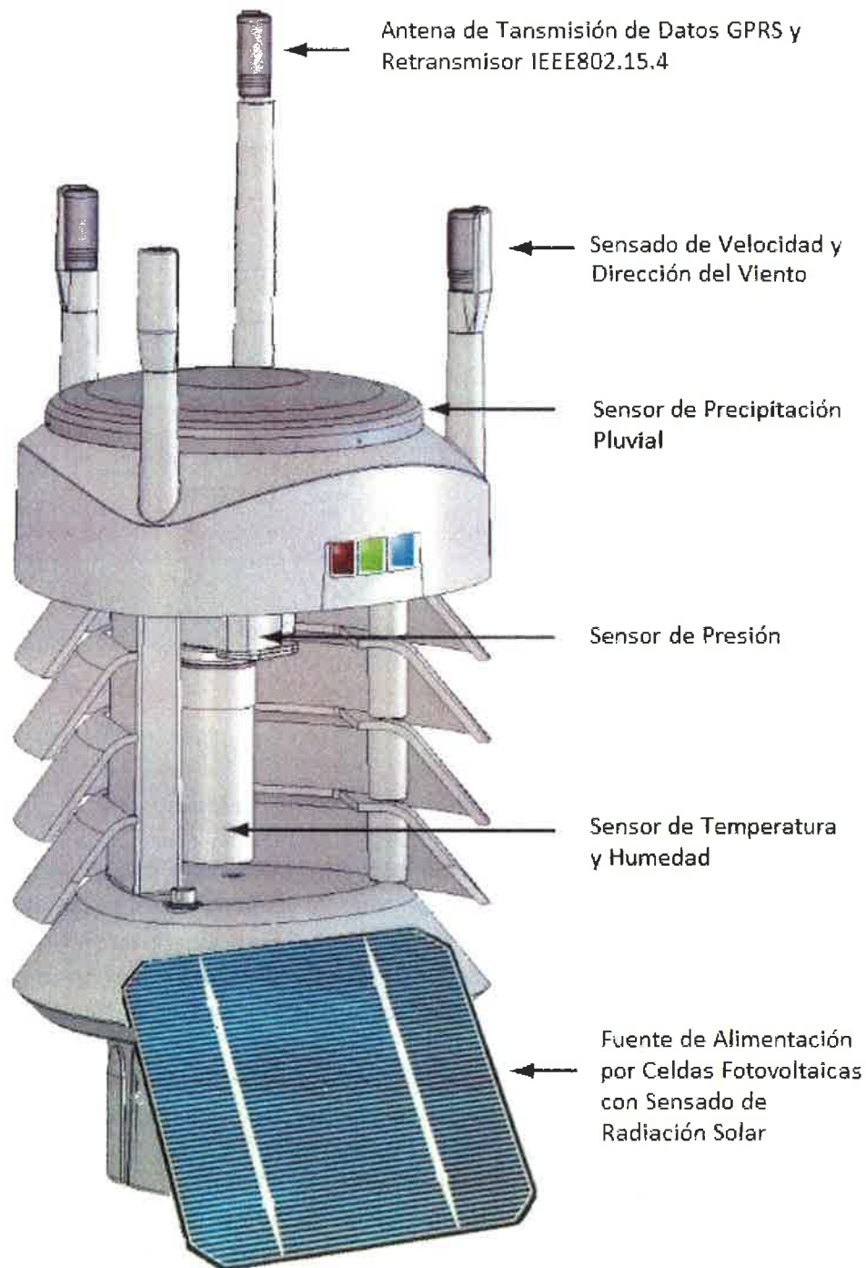
Figura 1 – Diseño conceptual preliminar del prototipo funcional Meteoromóvil.
