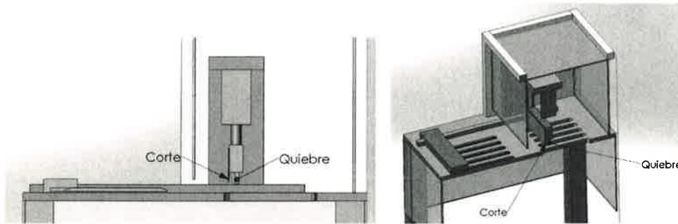
Ilustración 4, sistema de corte y quiebre.
