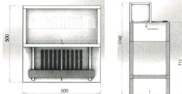
Ilustración 6, dimensiones conceptuales aproximadas (no se incluye la mesa).
